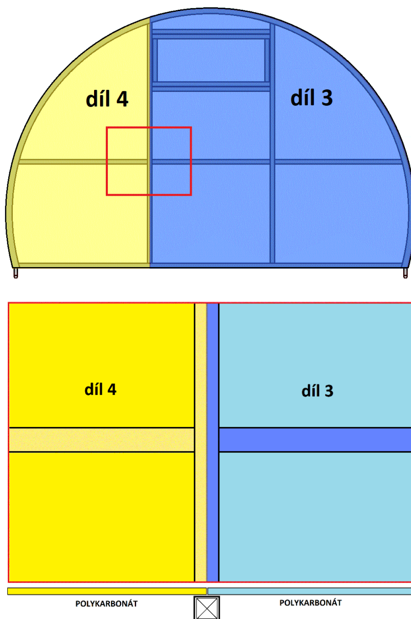
Obr. 7 – dva sousední díly 3 a 4 zarovnejte na střed svislého profilu
